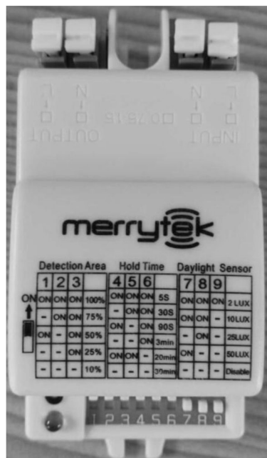
Dip-Schalter position
